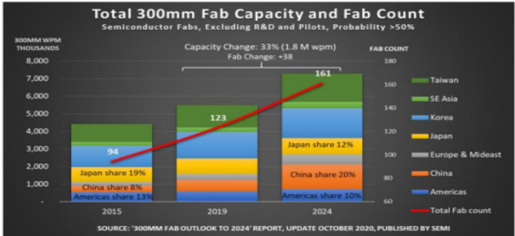
圖 2：2015 年、2019 年及 2024 年 12 吋晶圓廠總產能及總數走勢
